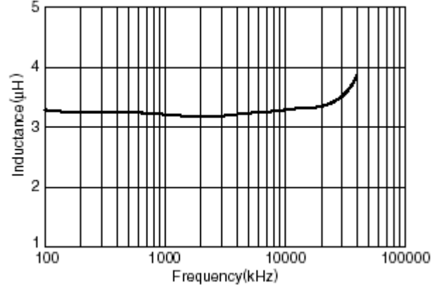
SDS5022M-3R3N-LF
