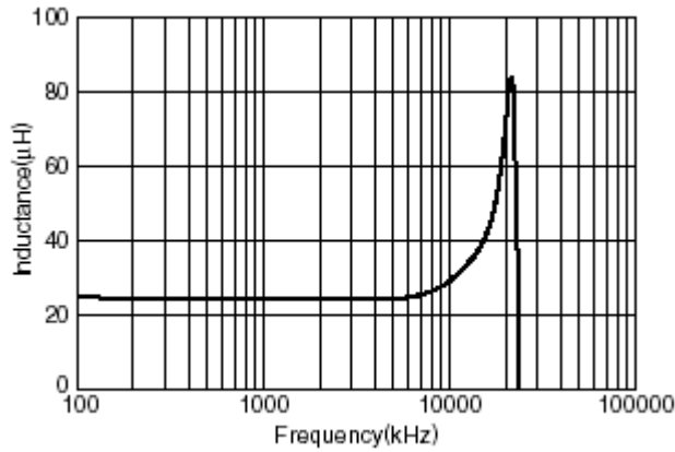
SDS5022M-220M-LF
