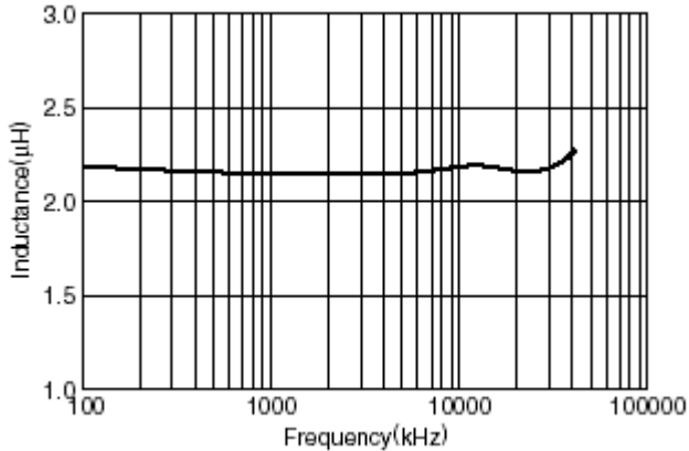
SDS5022M-2R2N-LF
